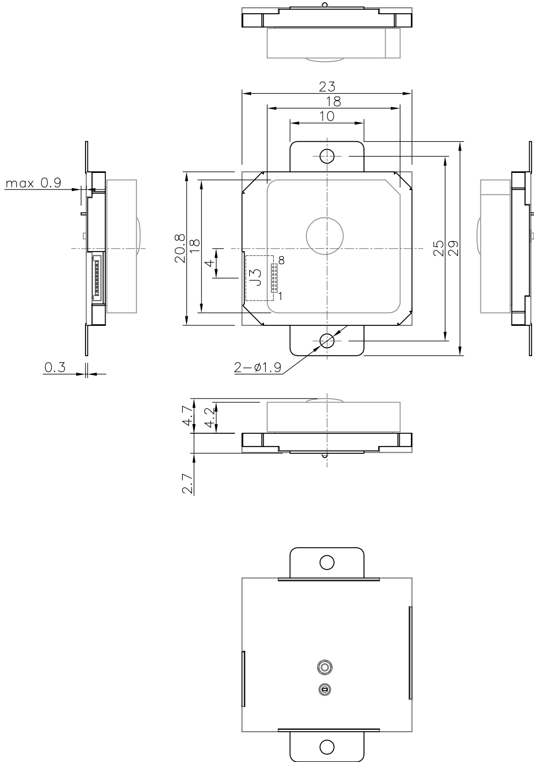
GPS-72A 外觀圖
